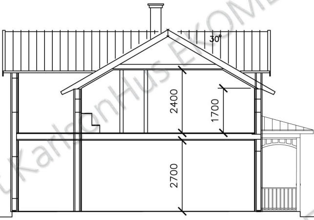
SEKTION
